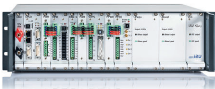
IAV Kivu Flexible Motorsteuerung
